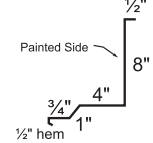
21. Side Chimney
