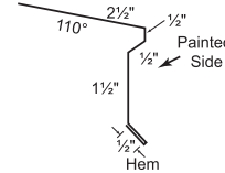
8. Drip Edge
