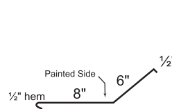
20. Bottom Chimney
