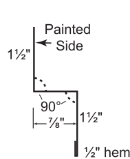
15. Double Angle
