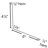
10A. Endwall
