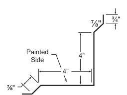
17. Eave Trim
